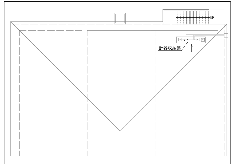
貯水槽上部平面図
