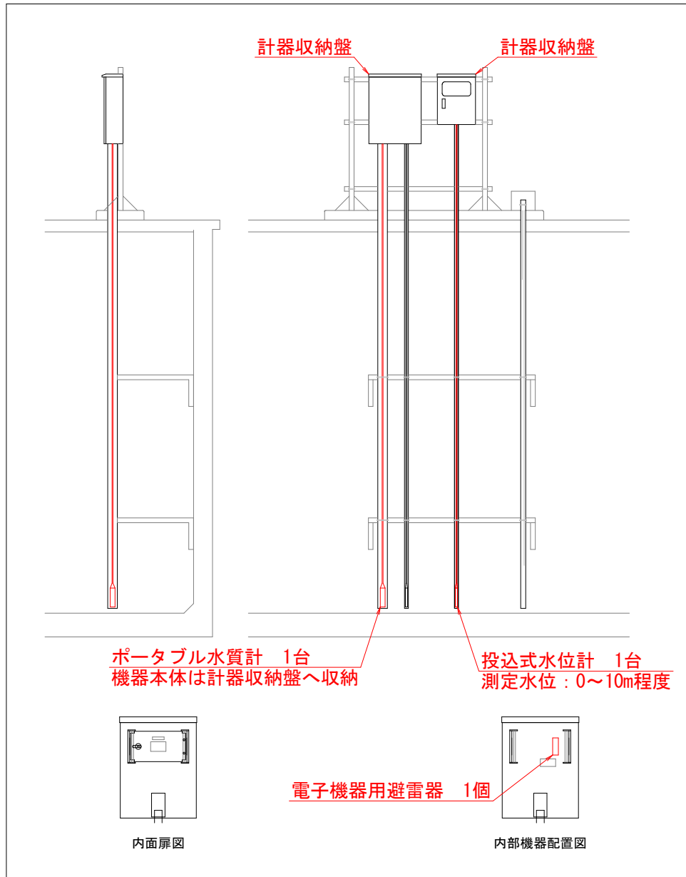
計器収納盤据付図
